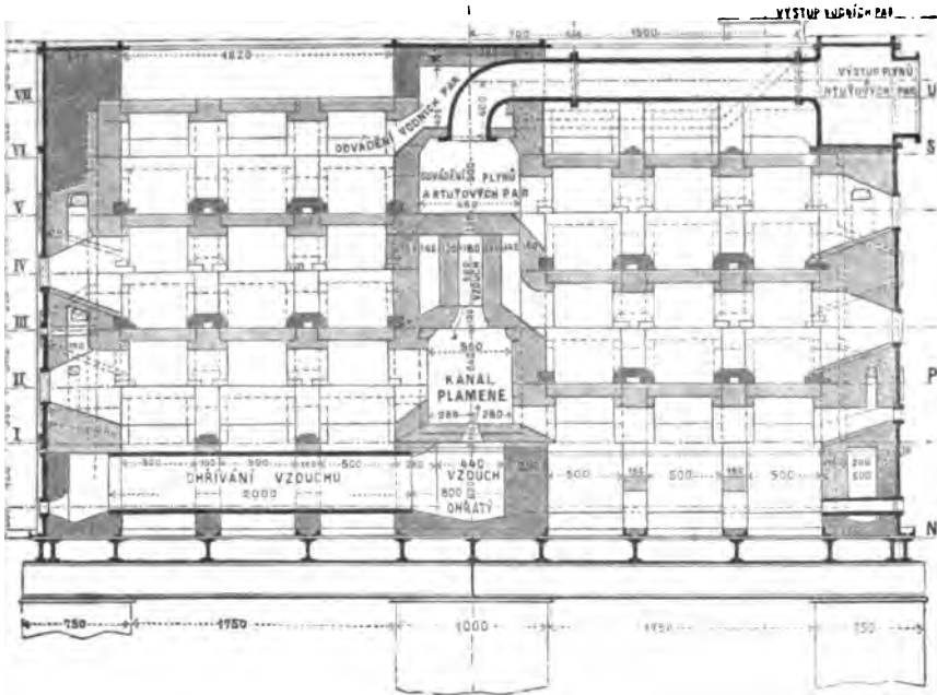
Řez příčný.
